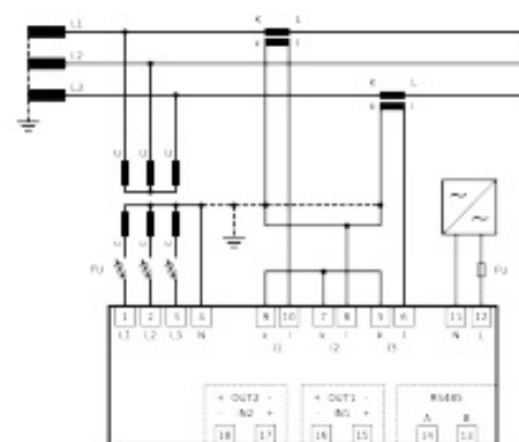
Podłączenie układ sieci s.n.
