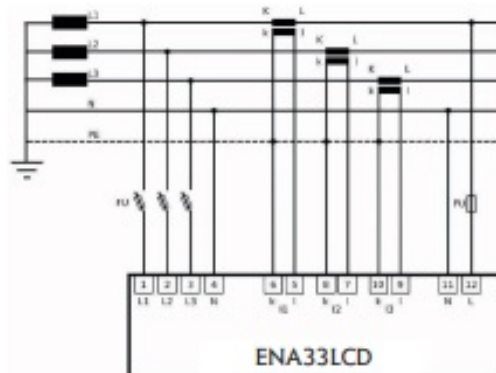
Pomiar 3-fazowy 4-przewodowy
