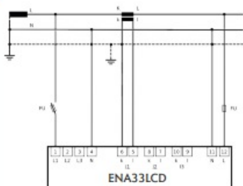
Pomiar 1-fazowy
