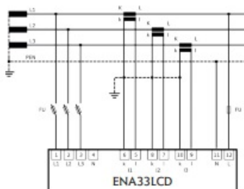
Pomiar 3-fazowy 3-przewodowy
