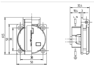
Zeichnung 1 MB 584 Maße in mm
