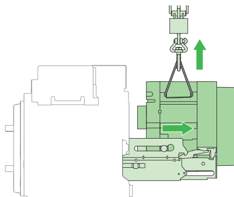
MTZ2/MTZ3
