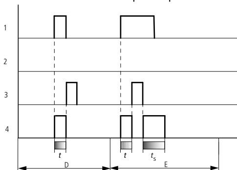
Obr. 151: Funkční diagram časového relé, podle impulsu 2
