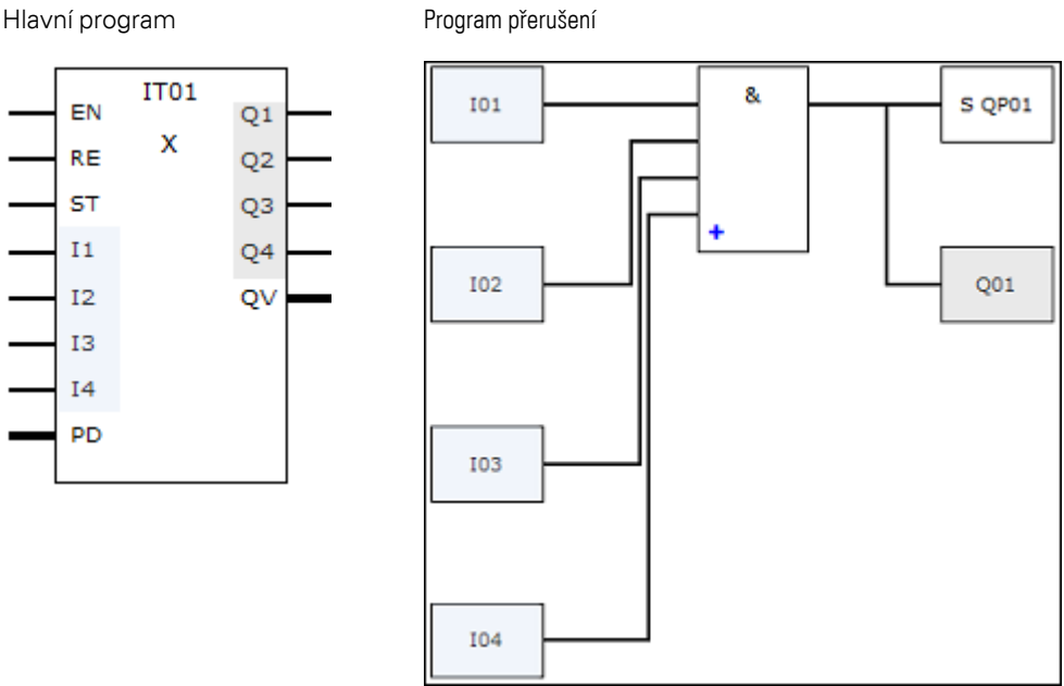
Obr. 269: Předání stavů ze vstupů a výstupů mezi hlavním programem a programem přerušení
