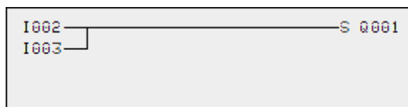
Obr. 116: Paralelní zapojení
