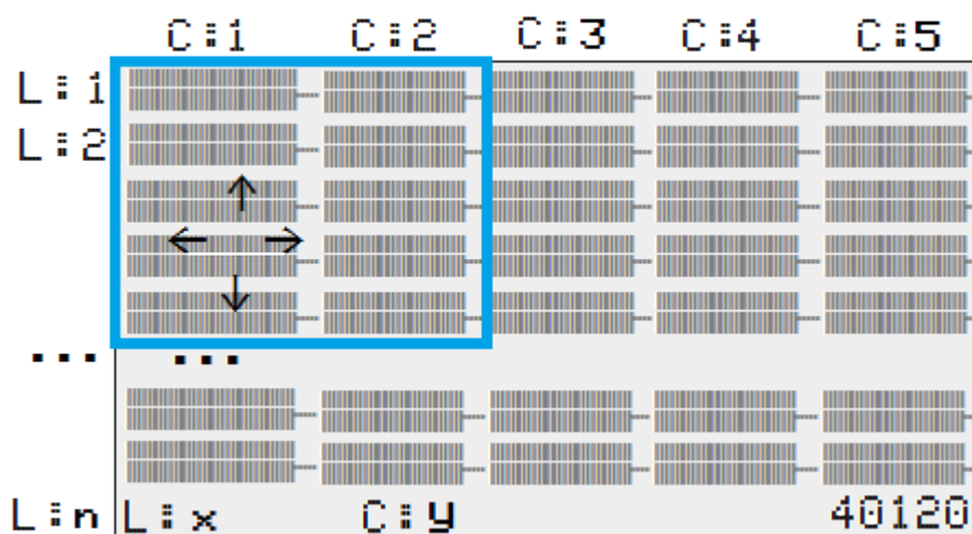
Obr. 82: Pole ve spínacím schématu
