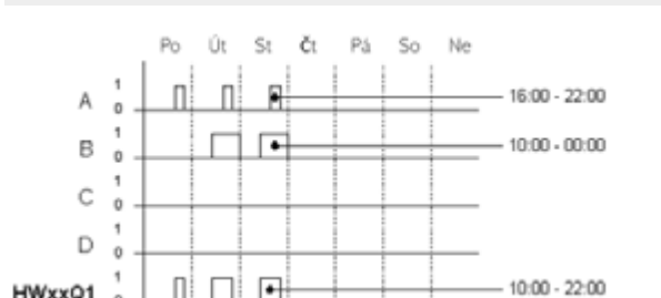
Obr. 132: Funkční diagram
