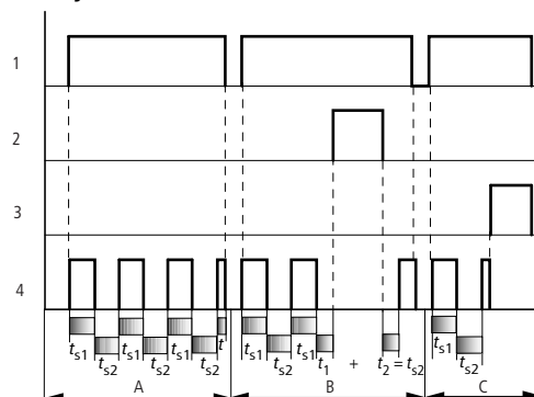
Obr. 152: Funkční diagram časového relé, podle impulsu
