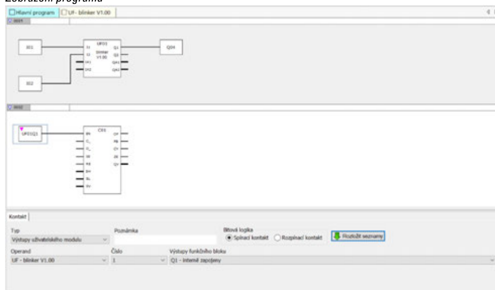
Obr. 279: Propojení vstupů/výstupů
