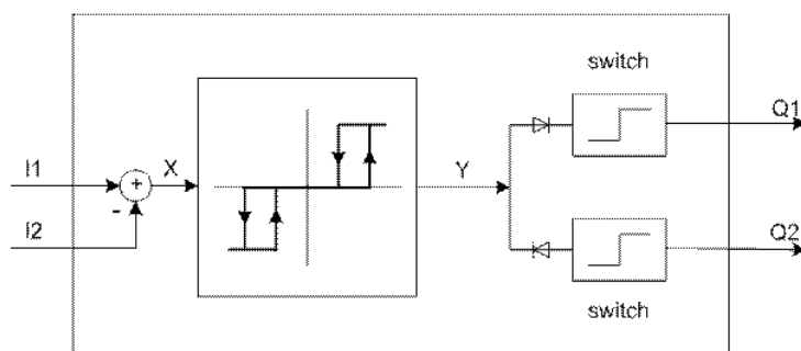
Obr. 203: Princip zapojení tříbodového regulátoru
