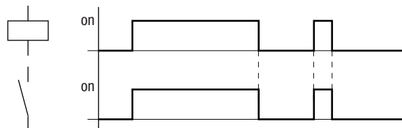
Obr. 97: Funkční diagram "Ochranná funkce"
