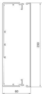
LF6023009010
