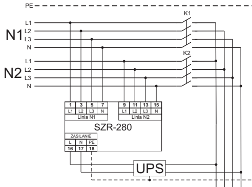
Rys. 12: Wykorzystanie wolnej linii jak źródła zasilania
