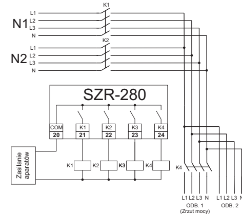
Rys. 13: Przykładowe podłączenie aparatów
