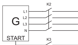
Rys. 4: Podłączenie generatora
