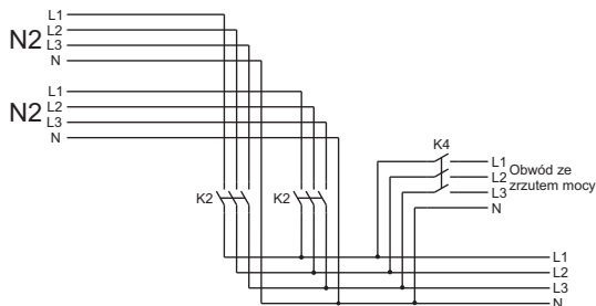
Rys. 2: Przykład obwodu ze zrzutem mocy
