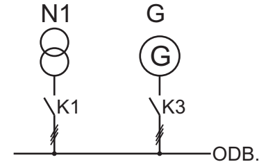
Rys. 8: Schemat obwodu dla programu N1 + G
