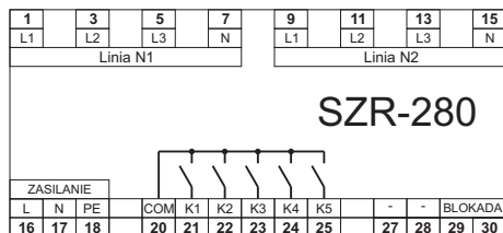
Rys. 10: Widok listwy zaciskowej sterownika SZR-280
