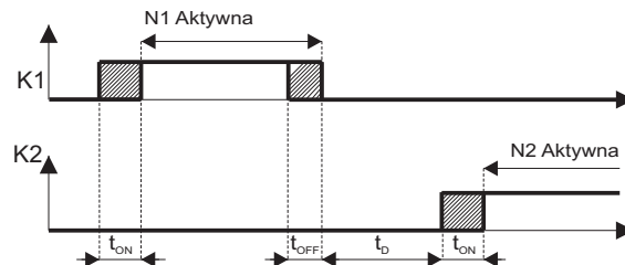
Rys. 6: Charakterystyka przełączenia linii
