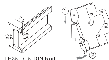
TH35-7.5 DIN Rail
