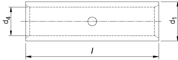
Crimp connector DIN 46267 bare
